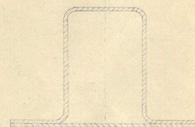
Schnitt C-C
