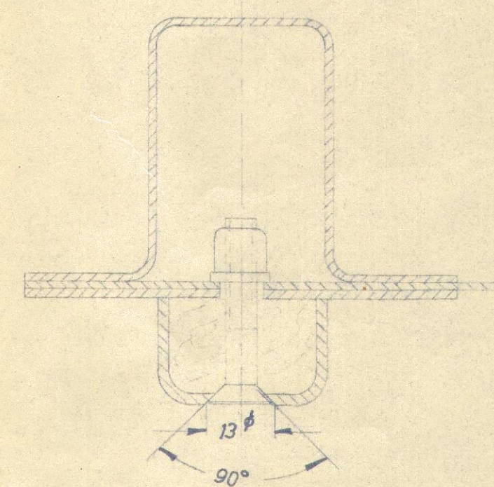
Schnitt A-A
